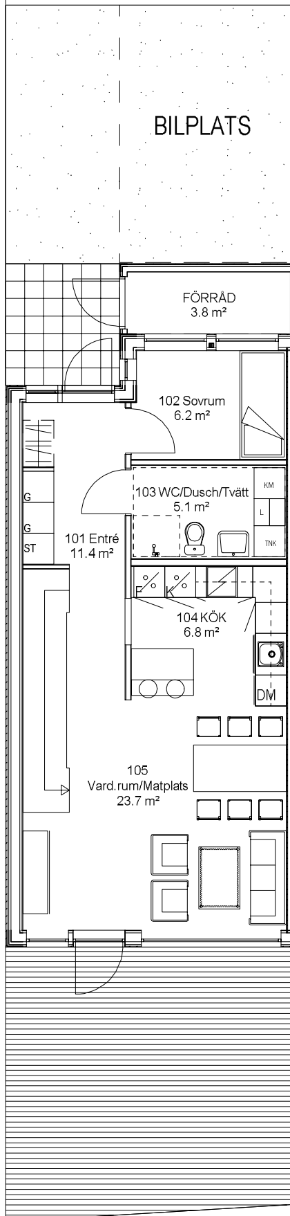
PLAN 1 - Rumshöjd 3000
