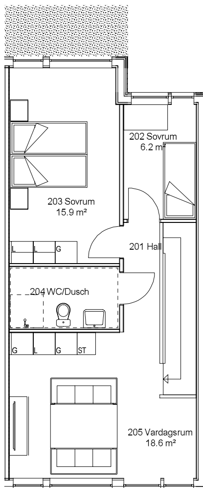
PLAN 2 - Rumshöjd 2700
